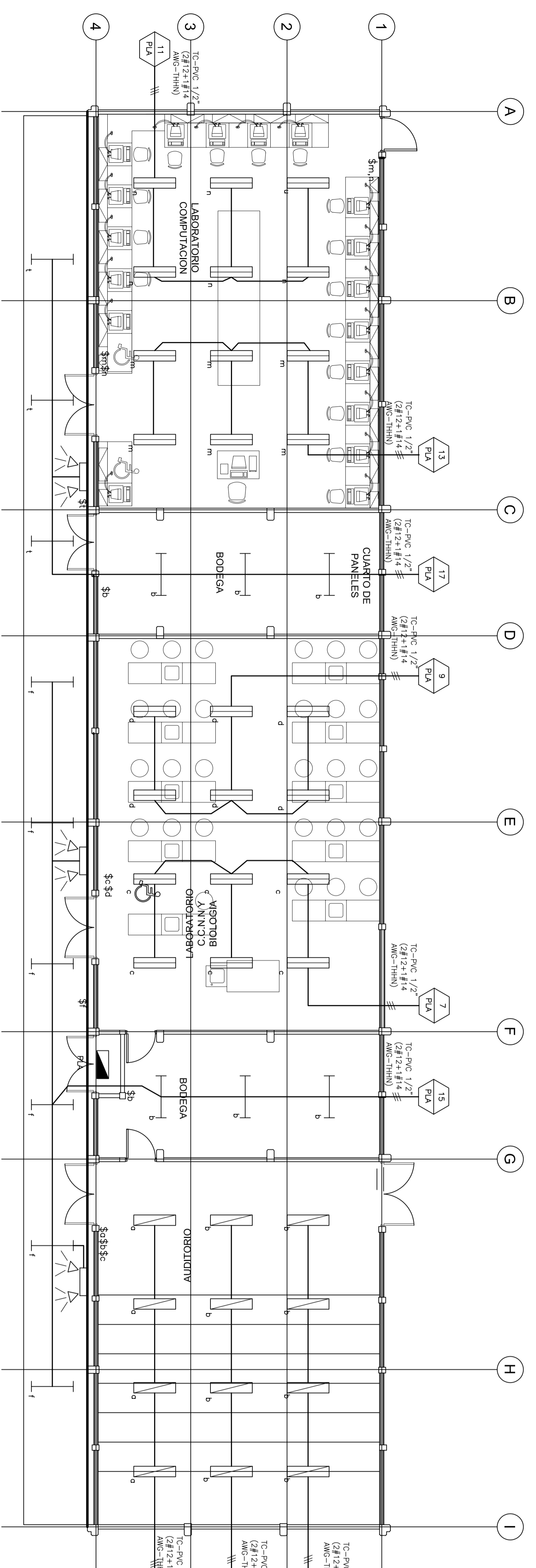
ILUMINACION DE EDIFICIO 5 LABORATORIO ESCALA 1 : 75
