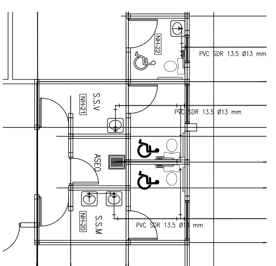
PLANTA DE AGUA POTABLE NH-20, NH-21 Y NH-22 ESCALA 1 : 75
