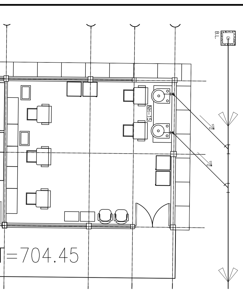
PLANTA DE AGUAS NEGRAS NH-15 ESCALA 1 : 75
