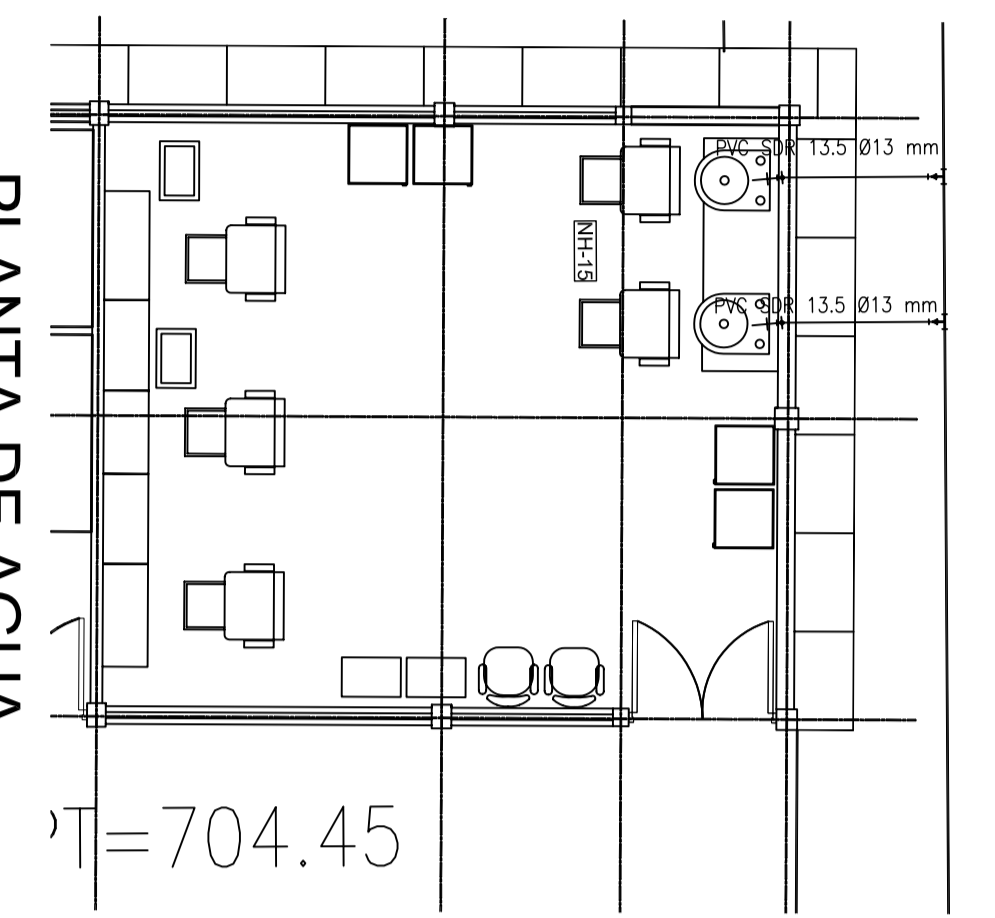
PLANTA DE AGUA POTABLE NH-15 ESCALA 1 : 75
