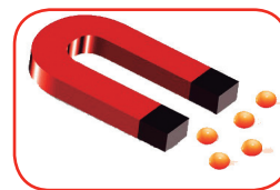
Imán
