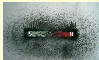
Campo magnético
